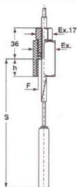
Conexión hembra, giratoria y deslizable.
