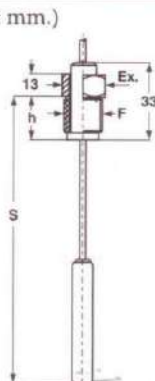
Conexión macho, giratorio.
