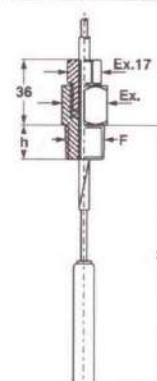
Conexión macho, giratorio y deslizable.
