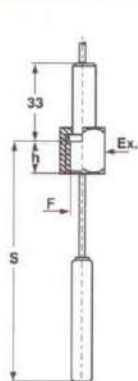
Conexión hembra, giratoria.
